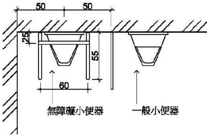
無障礙小便斗安裝圖說
